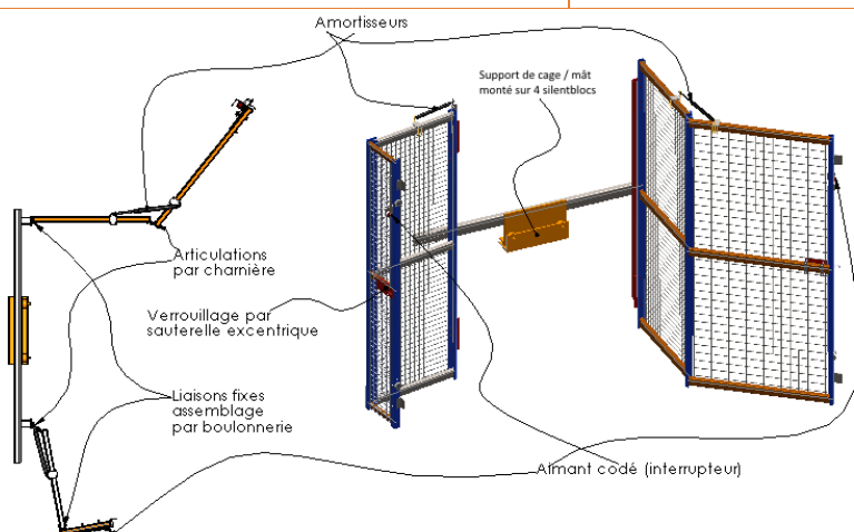
Cage de sécurité 2 vantaux double articulations
