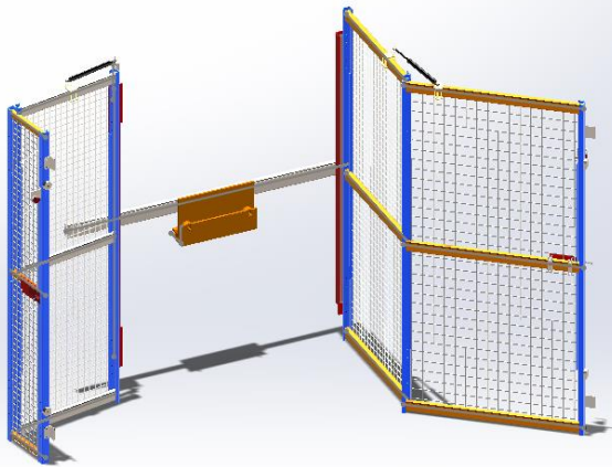
Cage de sécurité double ouverture
