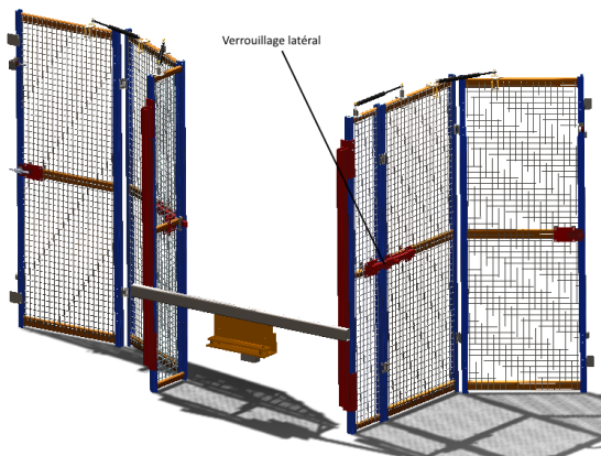
Cage de sécurité 2 vantaux double articulations
